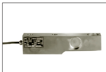
CELLULES À LA COUPE MOD. FT Capacités de 100 a 500 kg
