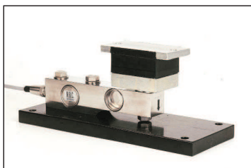
ACCESSOIRE POUR CELLULES MOD. FX Capacités de 1000 à 3000 kg
