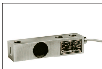
CELLULES À LA COUPE MOD. FB Capacités de 250 a 5000 kg
