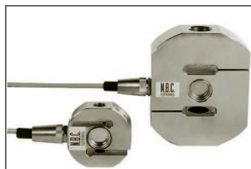
CELLULES À TRACTION MOD. SX Capacités de 150 a 10000 kg
